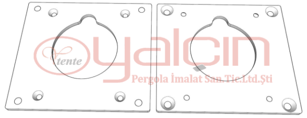
Dikme Üst Bağlantı Sacı / sewed top connection sheet PRG-02-10400-26-0X
