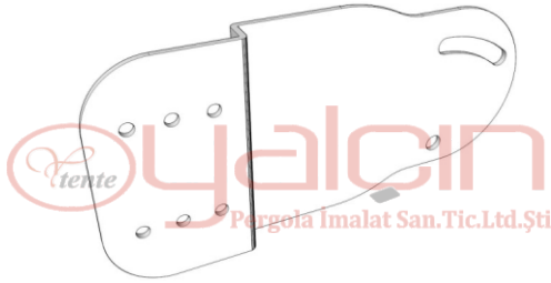
Arka Saç Deliklisiz Sol Bükümlü / Back sheet without hole left twisted PRG-02-10500-30-0X
