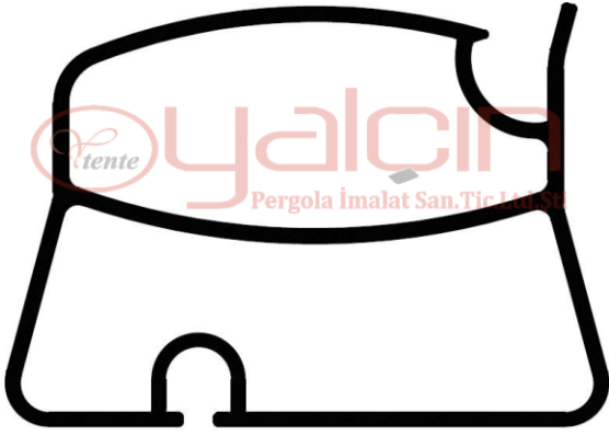
Büyük Kumaş Taşıyıcı Profili / Large Fabric Carrier Profile
