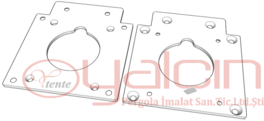
Dikme Üst Bağlantı Sacı / Sewed top connection sheet
