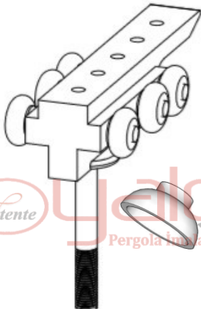
Büyük Kumaş Profil Arabası + Kapağı / Large Fabric Profile Trolley
