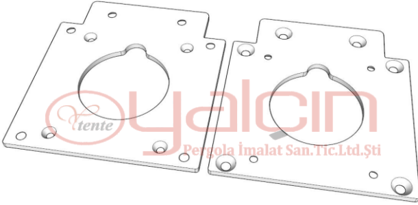
Dikme Üst Bağlantı Sacı / Sewed top connection sheet PRG-02-10400-31-0X
