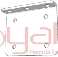
Ayak Üstü Bağlantı Sacı / Top leg connection
