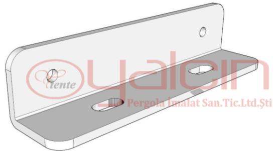
Trapez Bağlantı Sacı / Trapeze Connection Sheet PRG-02-10170-03-0X
